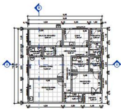
PLANTA BAIXA
